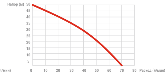
Насос поверхностный и насос-автомат 70/50
