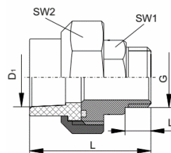
Рисунок 39. Муфта комбинированная разъемная (американка) с наружной резьбой
