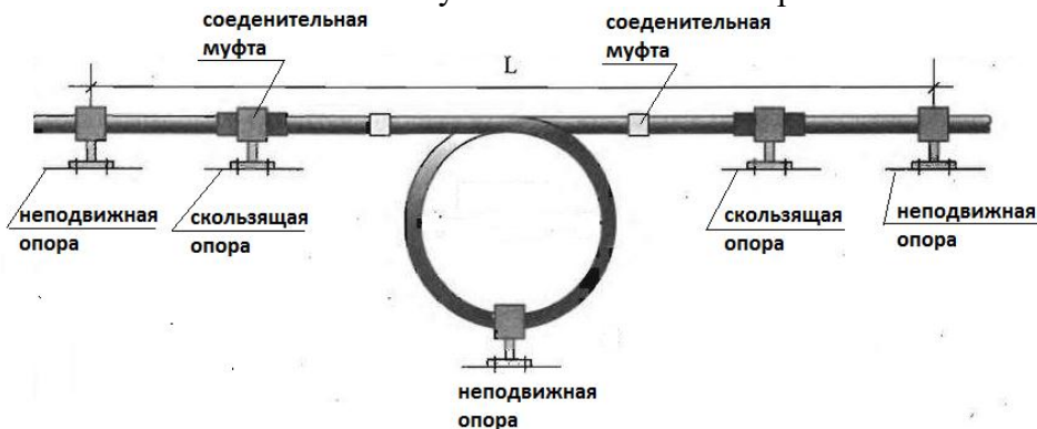
Рис. 3 схема установки компенсатора
