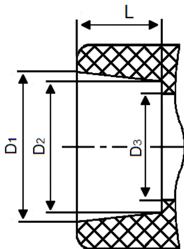
Рис 2. Раструбная часть фитингов серии PRO
