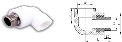
Рисунок 9. Угольник с наружной резьбой
