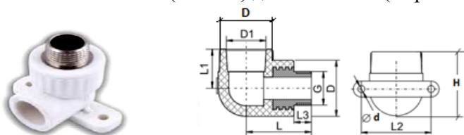
Рисунок 11. Угольник (особый) для смесителя (с креплениями) наружная резьба
