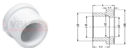
Рисунок 5. Бурт под американку
