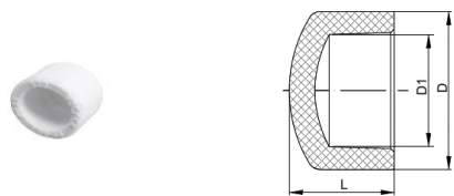
Рисунок 3. Заглушка
