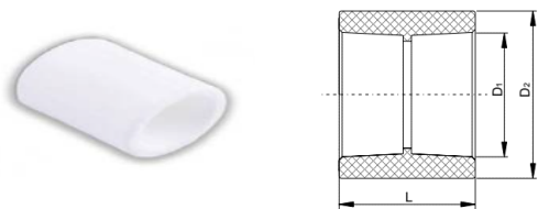
Рисунок 18. Муфта соединительная
