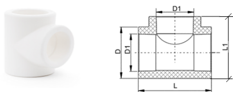
Рисунок 14. Тройник
