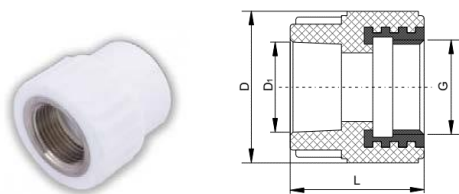
Рисунок 20. Муфта комбинированная с внутренней резьбой
