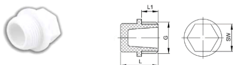
Рисунок 4. Заглушка резьбовая
