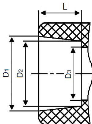
Рис 2. Раструбная часть фитингов серии PRO
