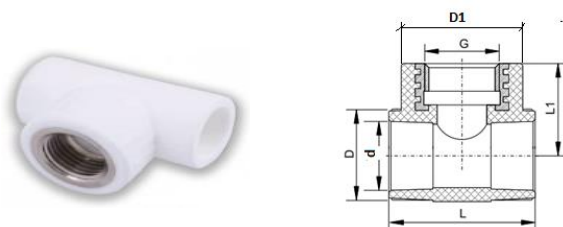
Рисунок 16. Тройник комбинированный с внутренней резьбой
