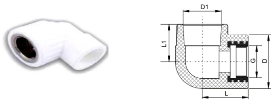
Рисунок 8. Угольник с внутренней резьбой
