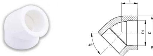
Рисунок 6. Угольник 45°
