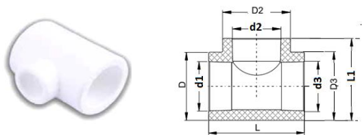
Рисунок 15. Тройник редуционный
