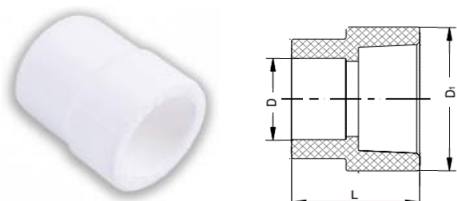
Рисунок 19. Муфта переходная ВН/НР
