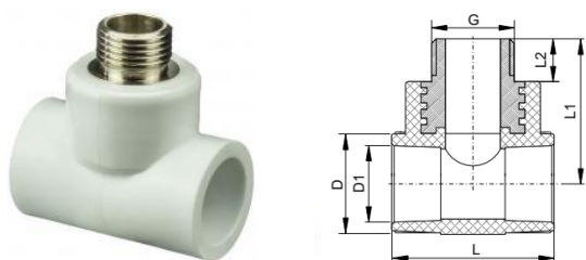
Рисунок 17. Тройник комбинированный с наружной резьбой
